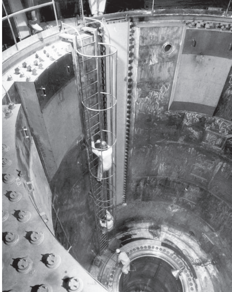
Ismerkedés a reaktortartállyal (1981)
